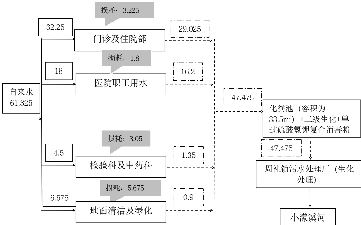
图3-1 周礼镇中心卫生院项目水平衡图 (m³/d)
