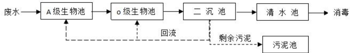
图 3-4 一体化设备废水处理工艺流程图
